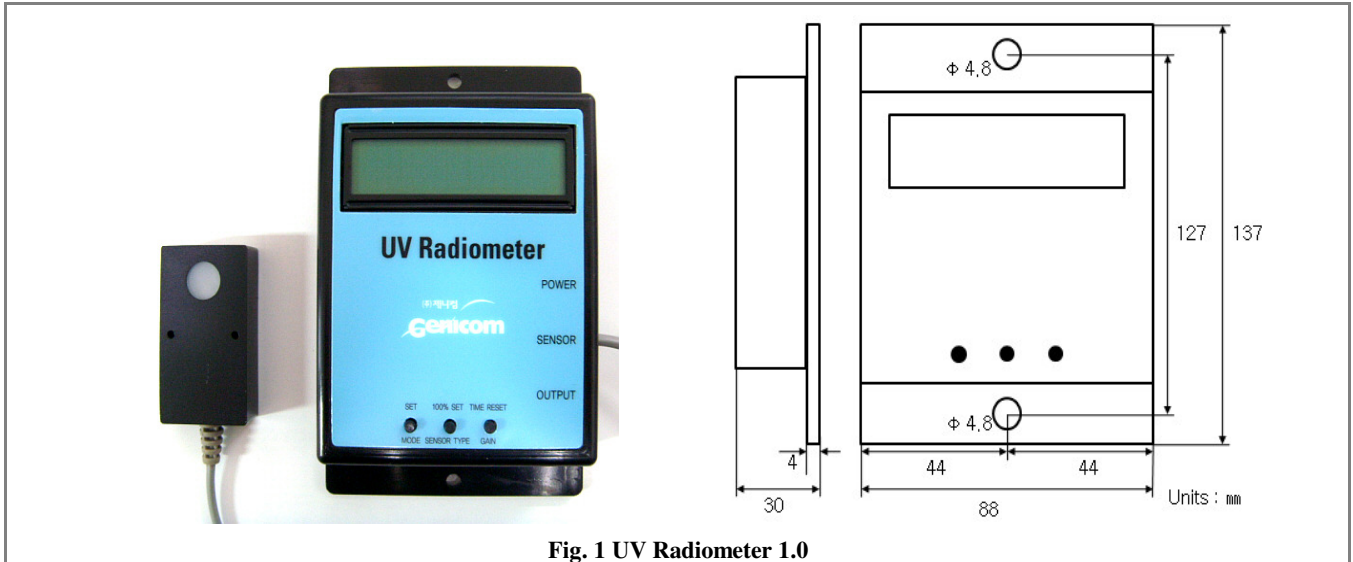
Fig. 1 UV Radiometer 1.0
